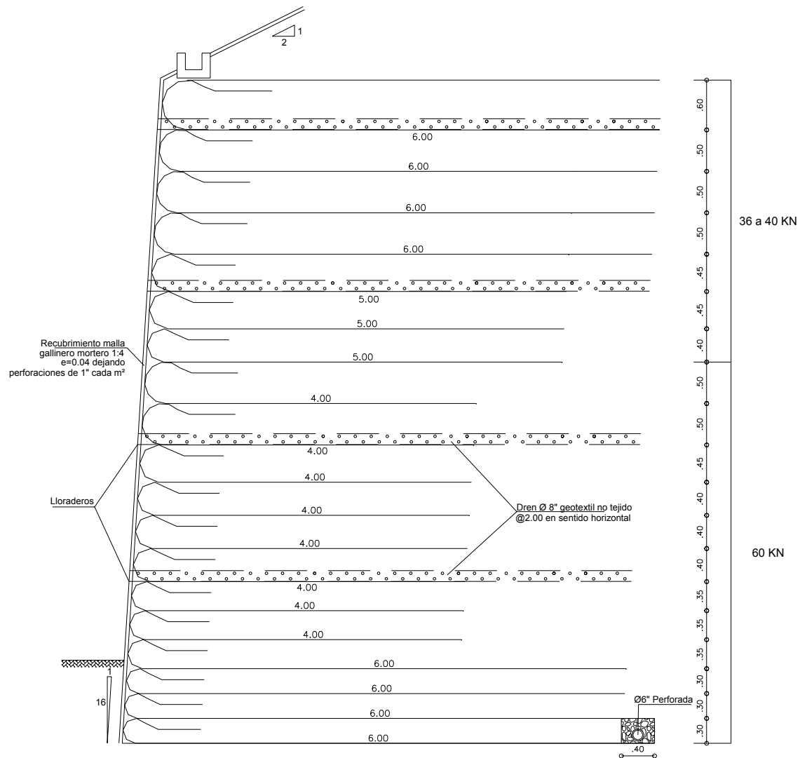
MURO h=8.00 1ª COMBINACIÓN Escala : 1 __ 50
