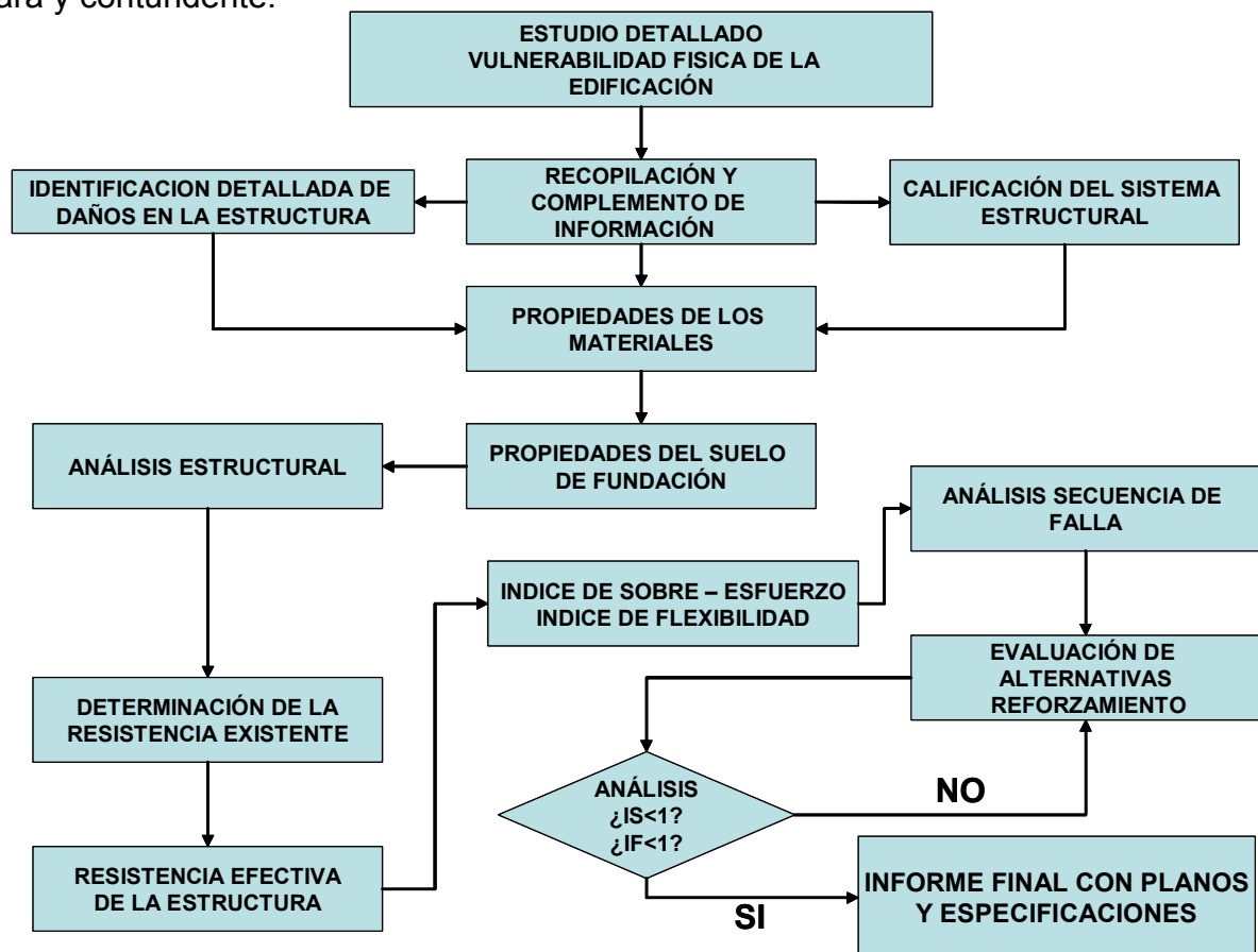
Gráfica 3. Esquema metodológico vulnerabilidad detallada
