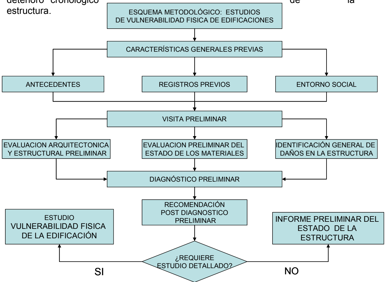
Gráfica 2. Esquema metodológico evaluación de vulnerabilidad preliminar.
